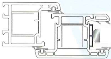
A-A Section
