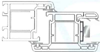
A-A Section
